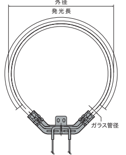
図-6 丸形仕様
