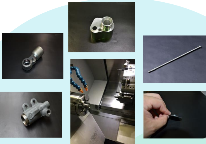
旋盤加工
